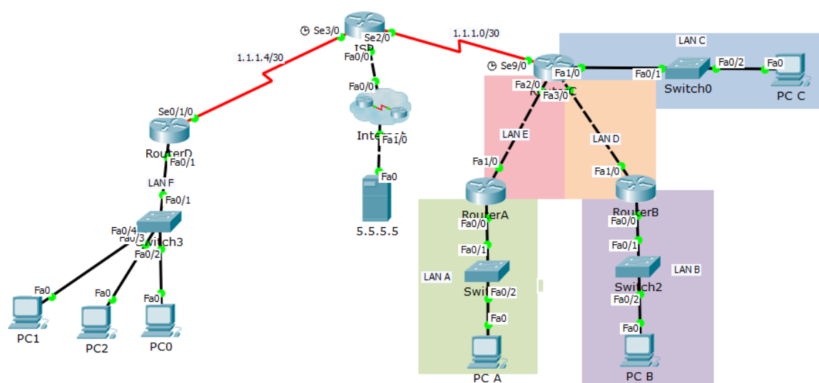
Рис. 1. Топология сети
